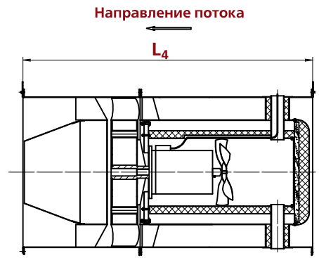
Компоновка 02
