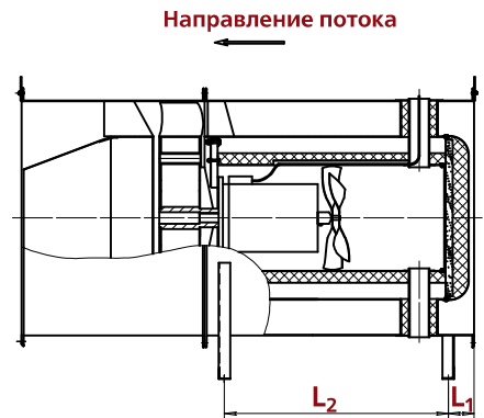
Компоновка 04
