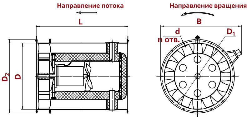
Компоновка 01
