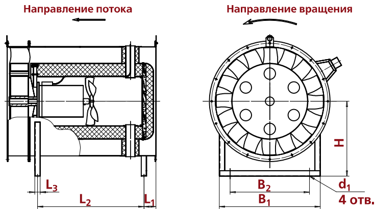
Компоновка 03
